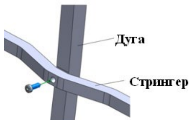
Узел 3. (Арка Стандартная)
